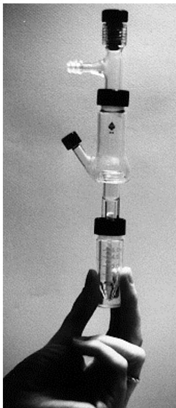
Figure 2 : Appareil à distillation muni d'une colonne à bande tournante pour séparer les constituants d'un mélange de volume compris entre 0,5 et 3 mL.
